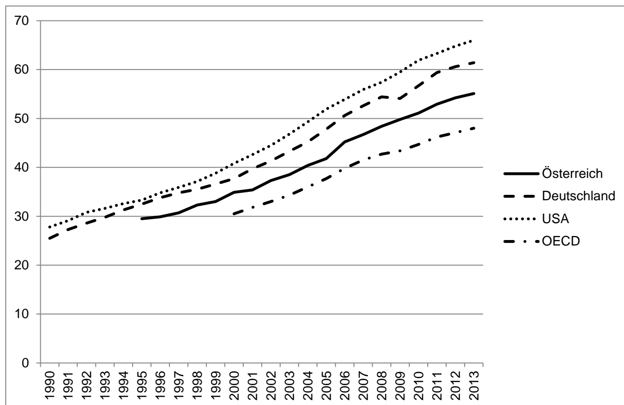
Abbildung 1: Arbeitsproduktivität, 1990-2013.
